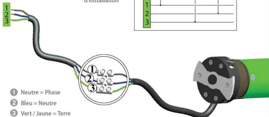
Schéma électrique d'installation
