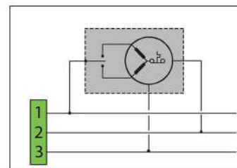
Schéma électrique d'installation
